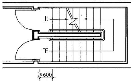
图 10 正对梯段设置的楼梯间门 距踏步边缘的最小安全距离示意图
